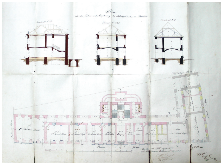
План зграде Ниже реалне гимназије, 1858.
